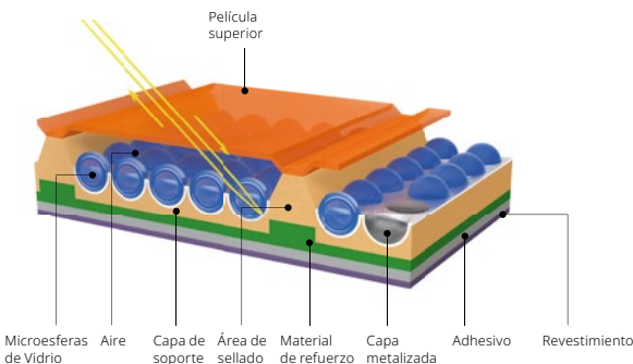
Fabricación Microesferas de Vidrio Encapsuladas
