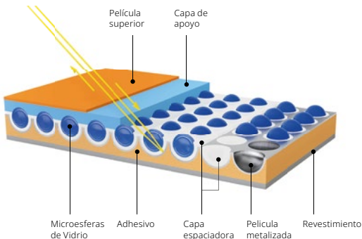
Fabricación Microesferas de Vidrio Incrustadas
